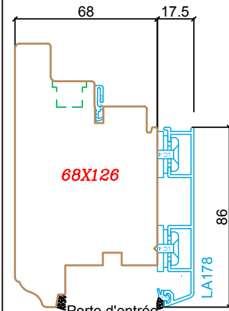
Porte d'entrée
