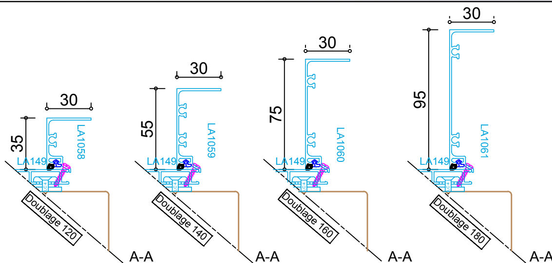
Tapées Alu
