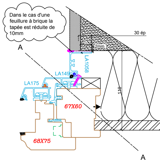
Tapée avec feuillure à brique
