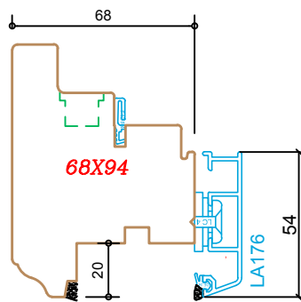
Traverse haute pour entrée d'air
