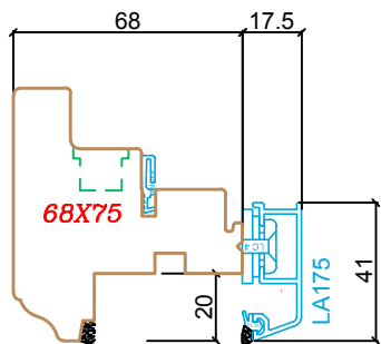
Fenêtre standard
