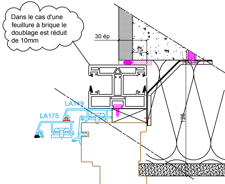
Coulisse avec feuillure à brique
