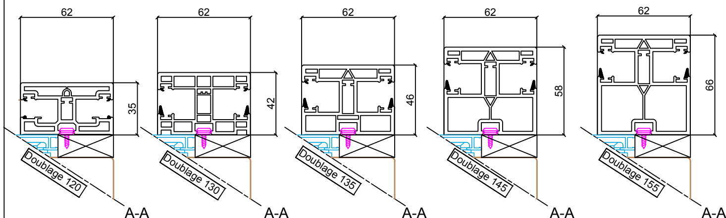
Seuil MACO
