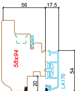
Traverse haute pour entrée d'air
