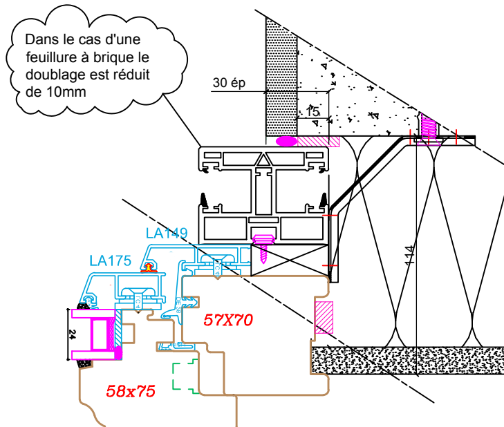
Coulisse avec feuillure à brique
