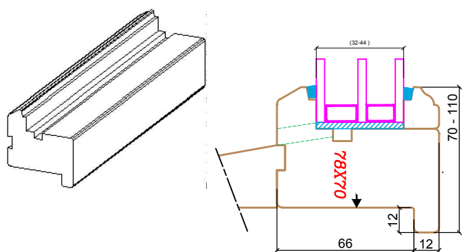
DORMANT "AILE A PLACO"
