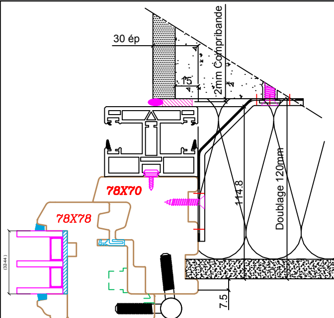
Coulisse avec feuillure à brique
