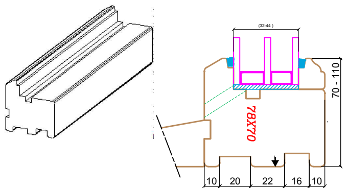
DORMANT "FEUILLURE A BRIQUE"
