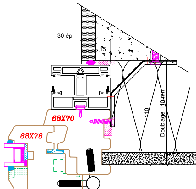
Coulisse avec feuillure à brique
