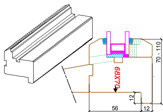
DORMANT "AILE A PLACO"
