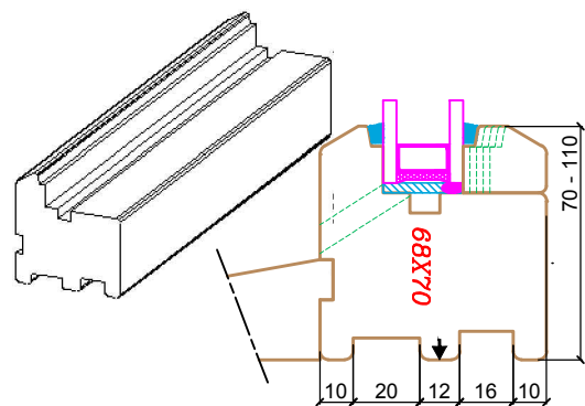
DORMANT "FEUILLURE A BRIQUE"
