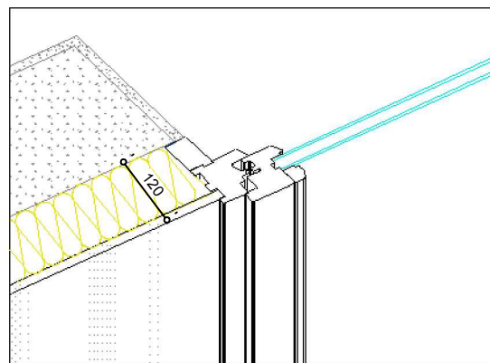
Detail feuillure à brique avec tapée
