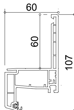
DORMANT Dréno 60
