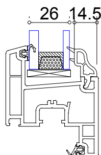
Vitrage 6-16-4
