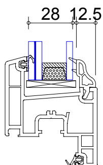
Vitrage 44.2-16-4
