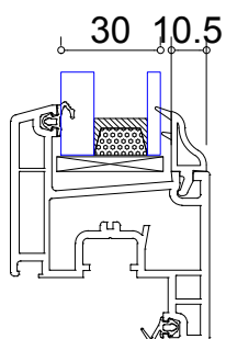
Vitrage 10-16-4
