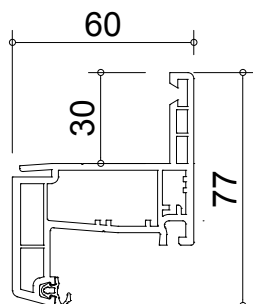
DORMANT Dréno 30
