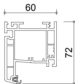
DORMANT D60VR
