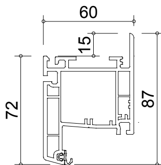
DORMANT D60
