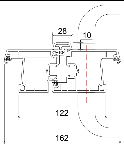
Battement en Z pour porte fenêtre (Z75BI) avec barillet
