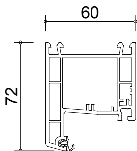
DORMANT D6
