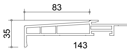
Appui 83 pour réno
