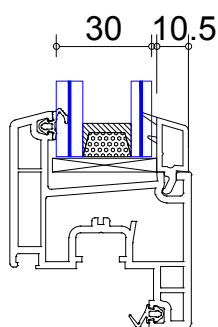
Vitrage 44.2-16-33.2
