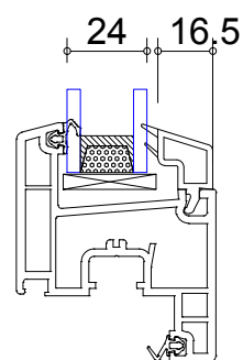
Vitrage 4-16-4
