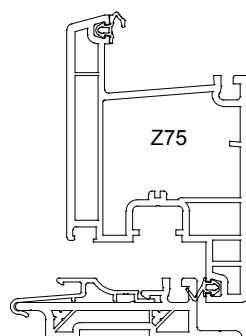
Seuil porte fenêtre
