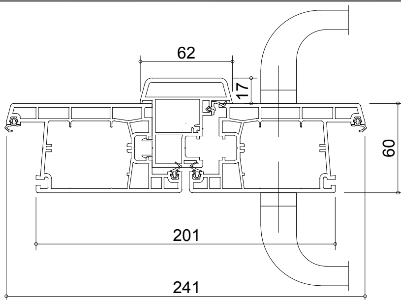
Battement en Z pour porte d'entrée (ZPEBI)
