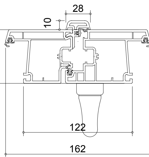
Battement en Z pour porte fenêtre (Z75BI) avec crémone
