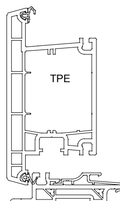
Seuil porte d'entrée (Profil en T)
