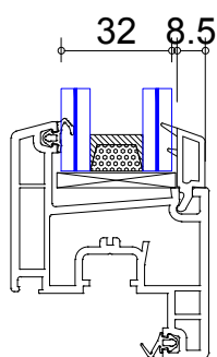
Vitrage 44.2-16-44.2
