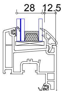
Vitrage 44.2-16-4
