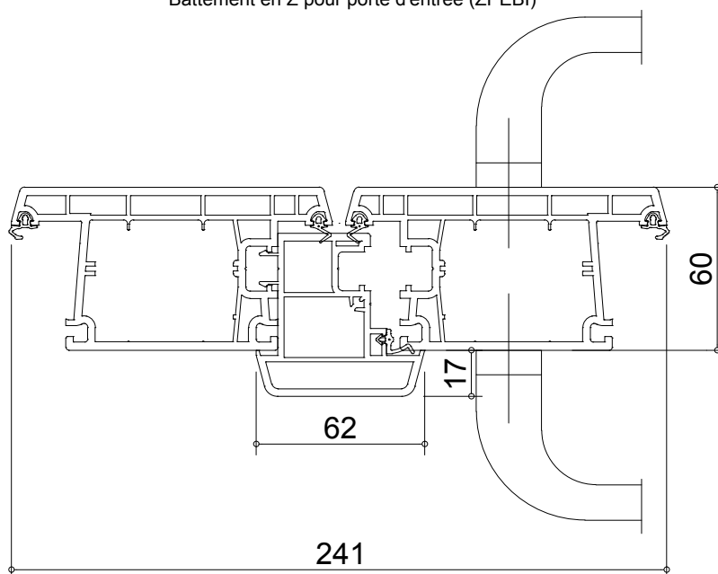
Battement en T pour porte d'entrée (TPEBI) Ouverture extérieure
