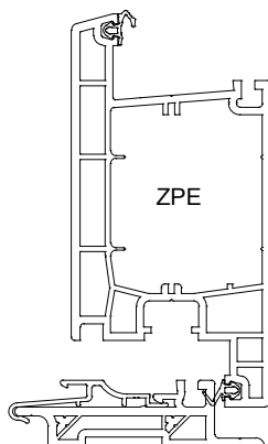
Seuil porte d'entrée (Profil en Z)
