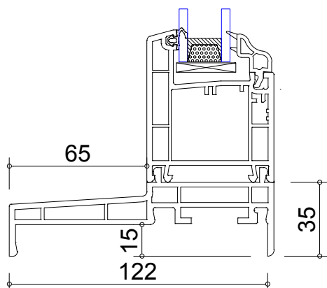
Appui 125 pour D6
