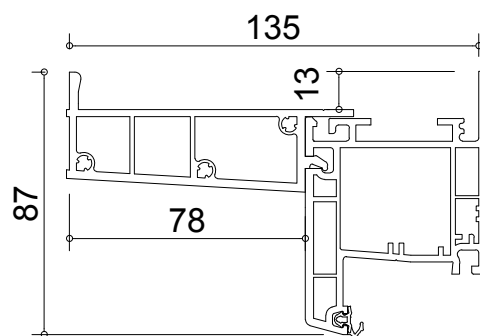
tapée de 78 + D60
