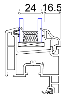
Vitrage 4-16-4
